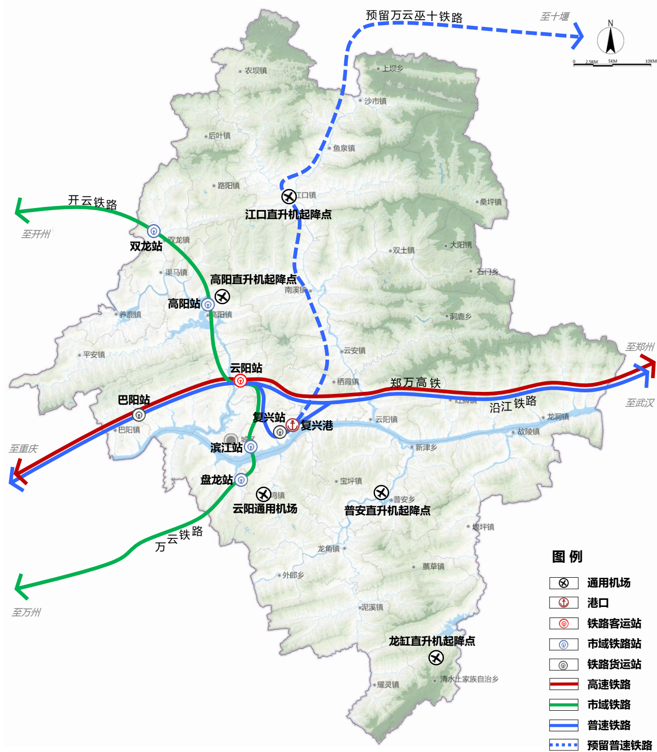
县域铁路、机场、港口规划图
