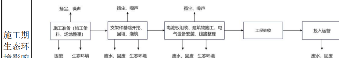
图 4.1-1 施工工艺流程和产排污节点图
