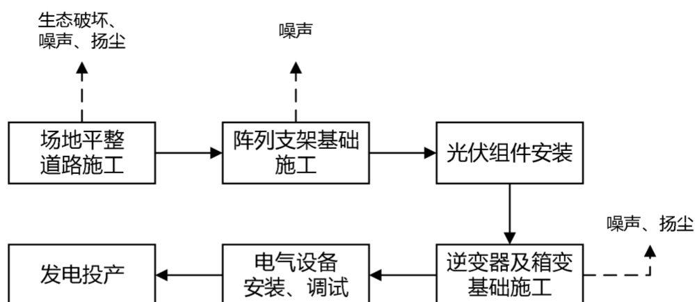
图 2.5-1 本项目施工工艺图
