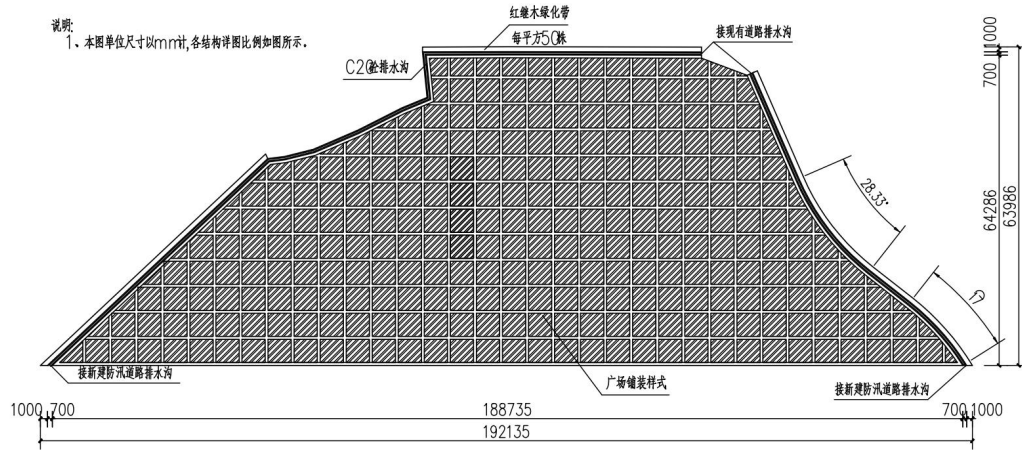
图 2.5.2-2 亲水广场（1#附属广场）大样图
