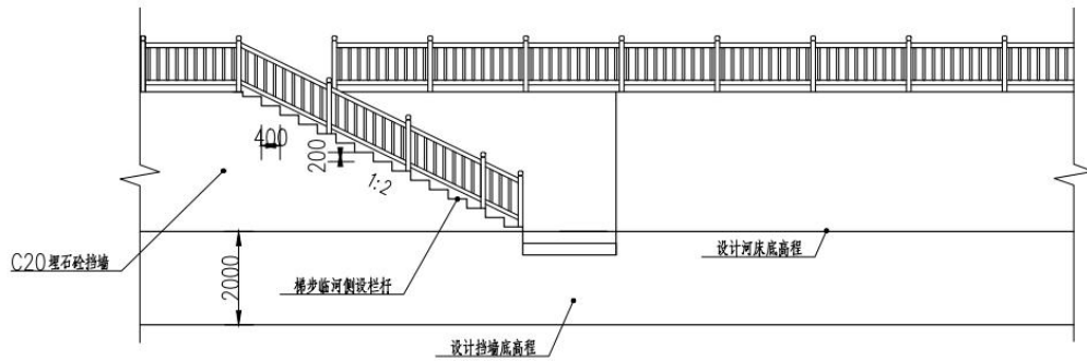
图 2.5.2-6 下河梯步大样图
